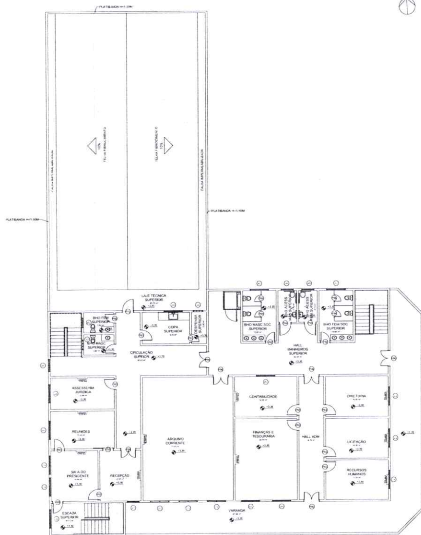
1 PAVIMENTO SUPERIOR ESCALA 1:100
