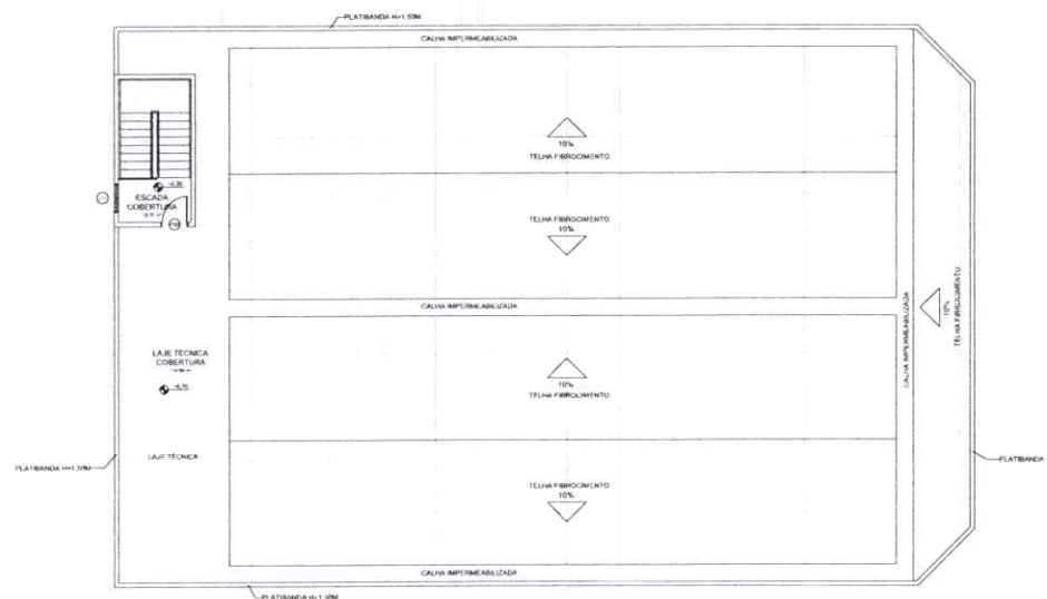
2 COBERTURA ESCALA 1:100
